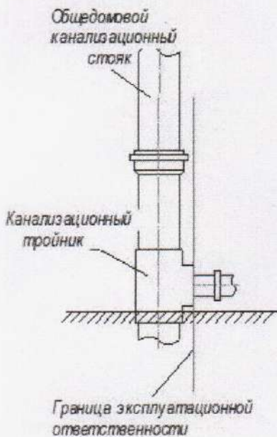
Рис. 3 Система водоотведения
