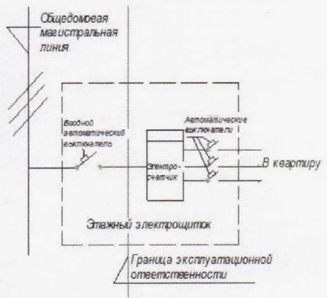
Рис. 4 Система электроснабжения
